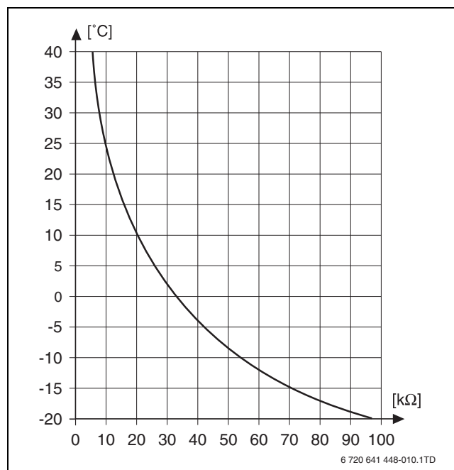
Rys. 11 Charakterystyka rezystancji dla czujników temperatury zewnętrznej
