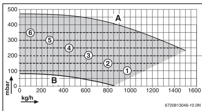
Rys. 8 Ciśnienie dyspozycyjne pompy przy GB192-35 i
