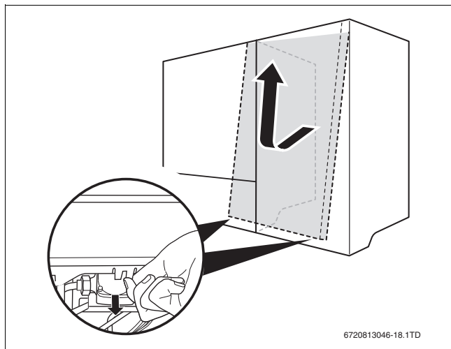
Rys. 18 Demontaż obudowy zasobnika warstwowego c.w.u.
