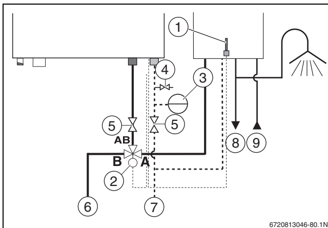
Rys. 27 Montaż zewnętrznego zaworu 3-drogowego (230 V)
