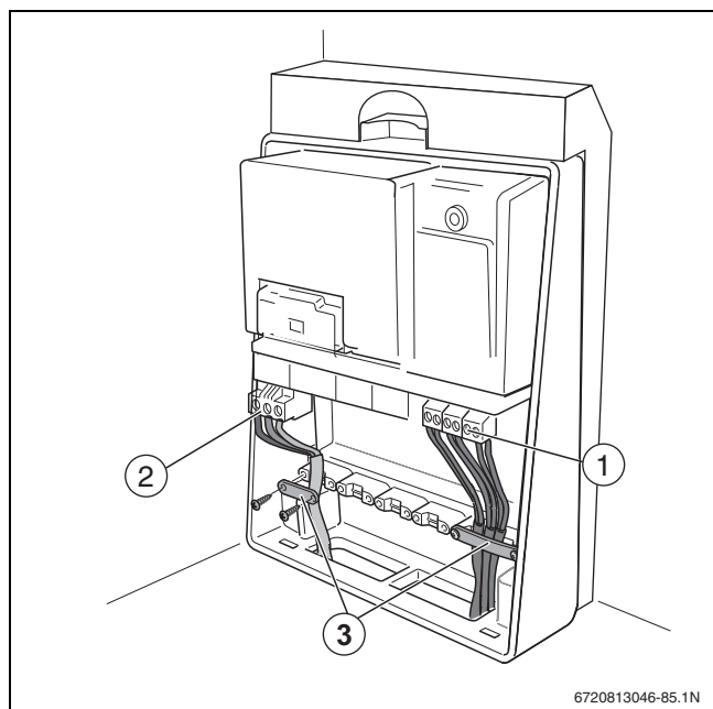
Rys. 35 Montaż opaski zaciskowej
