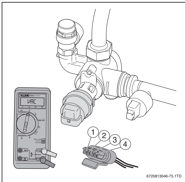
Rys. 63 Zawór 3-drogowy
