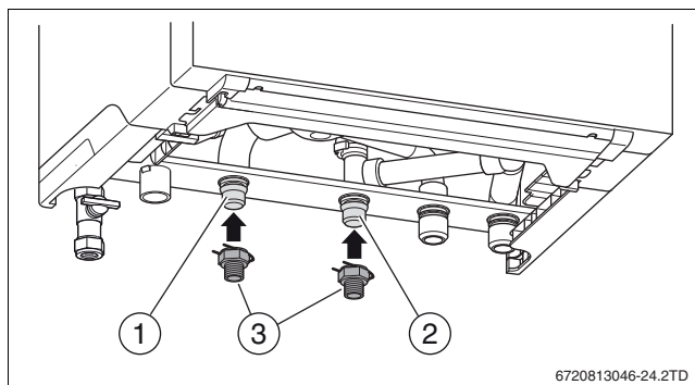
Rys. 24 Montaż przewodów rurowych dla zewnętrznego podgrzewacza pojemnościowego c.w.u.
