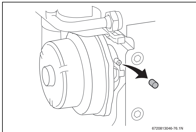
Rys. 59 Króciec pomiarowy na urządzeniu mieszającym
