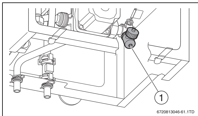
Rys. 52 Opróżnianie podgrzewacza pojemnościowego c.w.u. T40S
