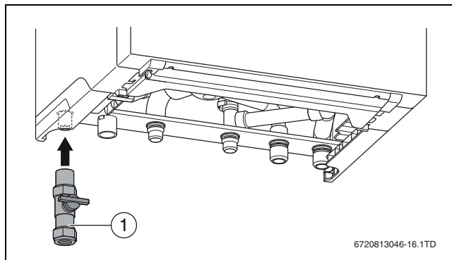
Rys. 16 Wykonanie przyłącza gazowego
