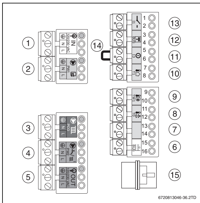
Rys. 33 Listwy zaciskowe
