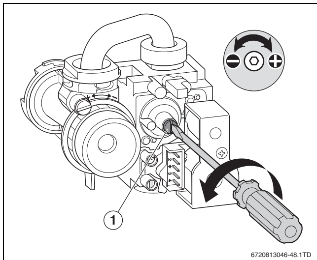
Rys. 43 Wykręcanie śruby
