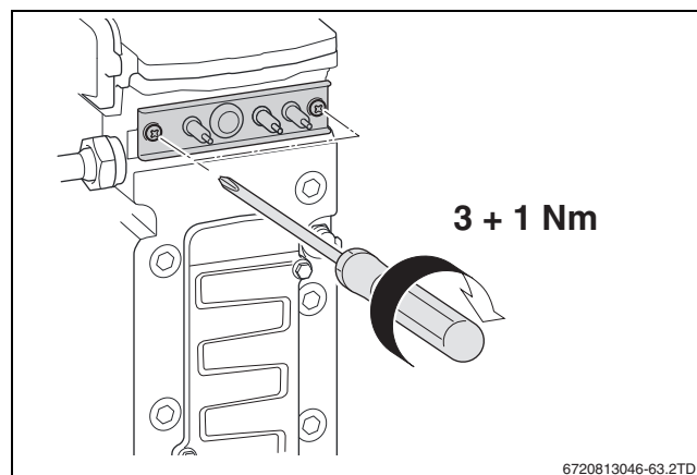
Rys. 53 Montaż zestawu elektrod
