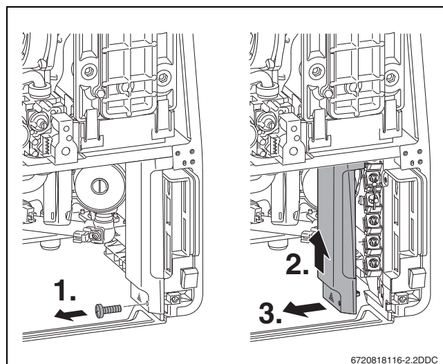
Rys. 32 Pokrywa zacisków przyłączeniowych
