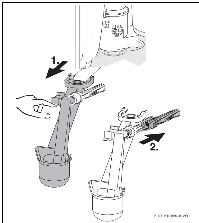
Rys. 58 Syfon kondensatu
