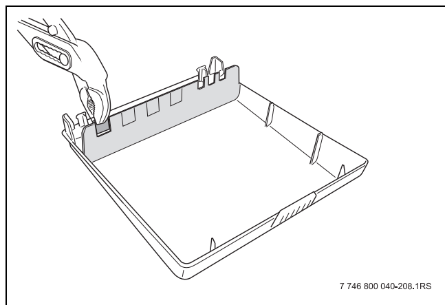
Rys. 36 Wyłamanie przepustu kablowego
