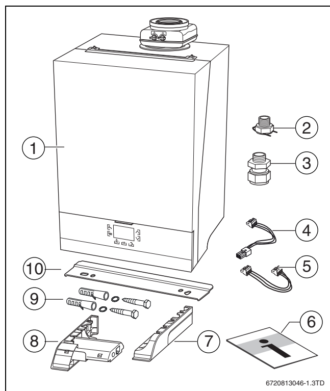
Rys. 1 Zakres dostawy
