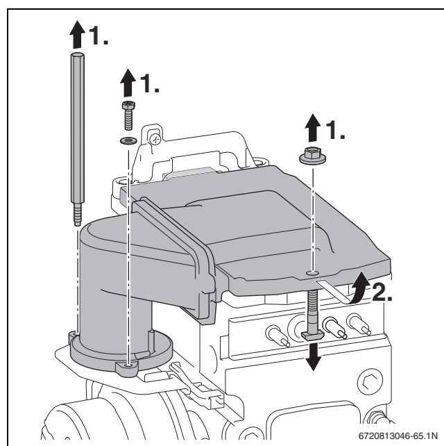
Rys. 55 Demontaż pokrywki palnika
