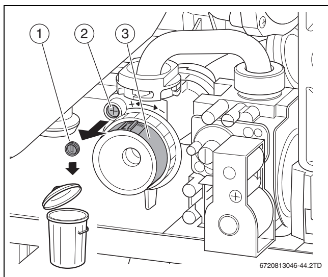
Rys. 41 Zdjęć plombę
