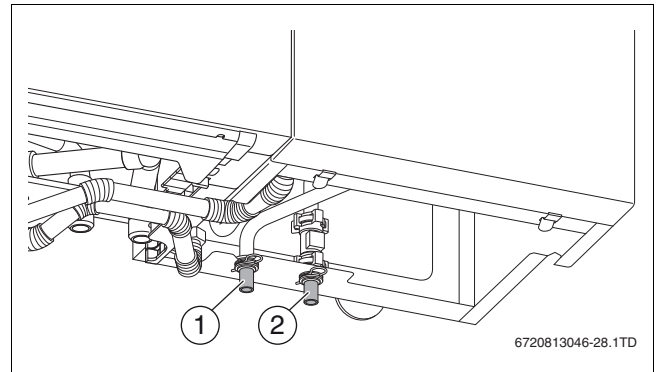
Rys. 28 Przyłącza wody
