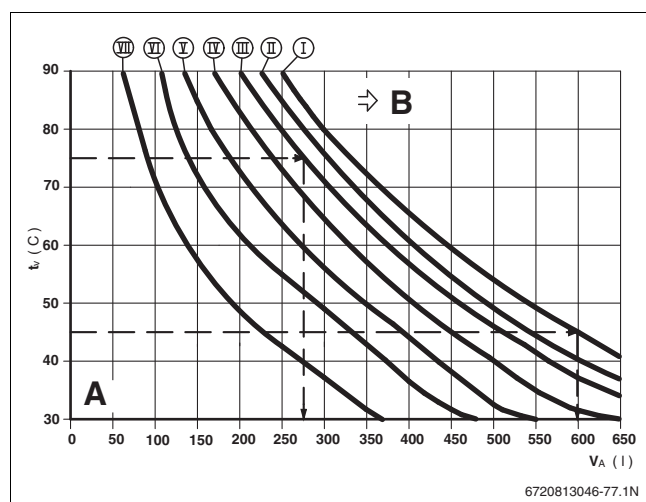
Rys. 23 Sprawdzić charakterystyki naczynia wzbiorczego, naczynia wzbiorczego c.o. 15 l
