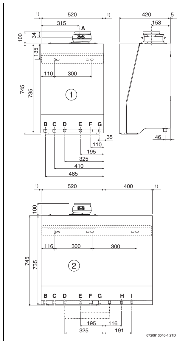
Rys. 5 Wymiary i przyłącza [mm]
