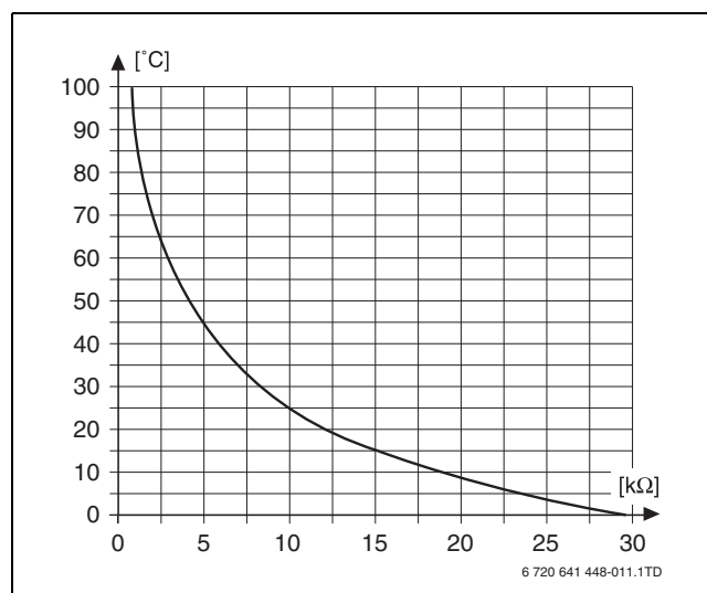
Rys. 10 Charakterystyka rezystancji czujników temperatury (nie dotyczy czujników temperatury zewnętrznej)
