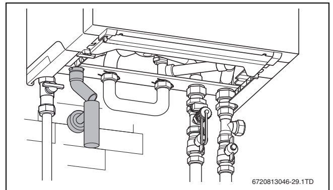
Rys. 29 G-TA Syfon kondensatu (osprzęt)
