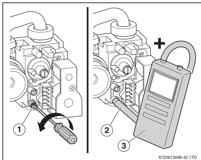
Rys. 40 Pomiar ciśnienia gazu na przyłączy
