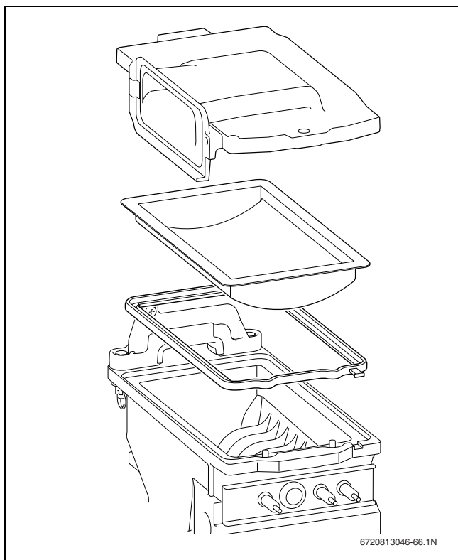
Rys. 56 Wymywanie palnika
