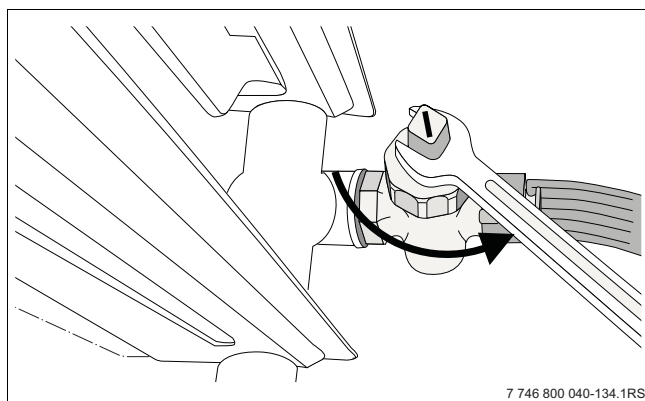
Rys. 51 Spuszczanie wody z instalacji ogrzewczej, gdy istnieje niebezpieczeństwo zamarznięcia
