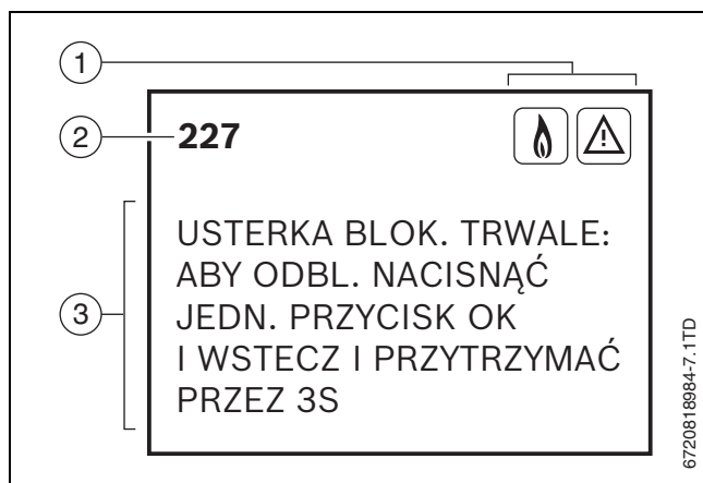
Rys. 64 Menu usterek
