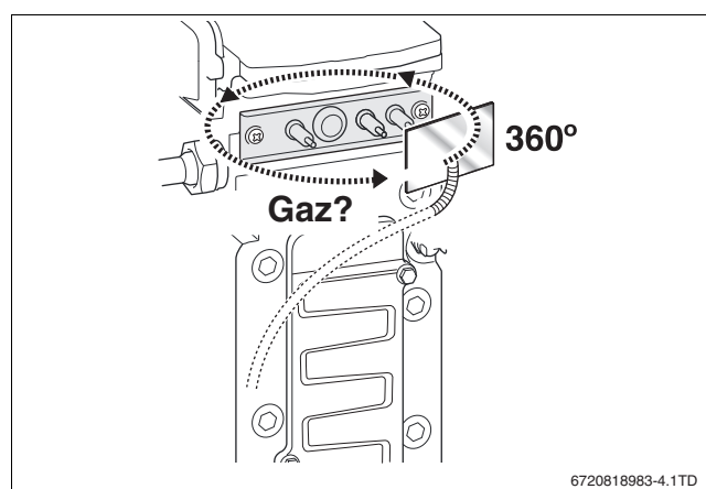
Rys. 54 Próby szczelności
